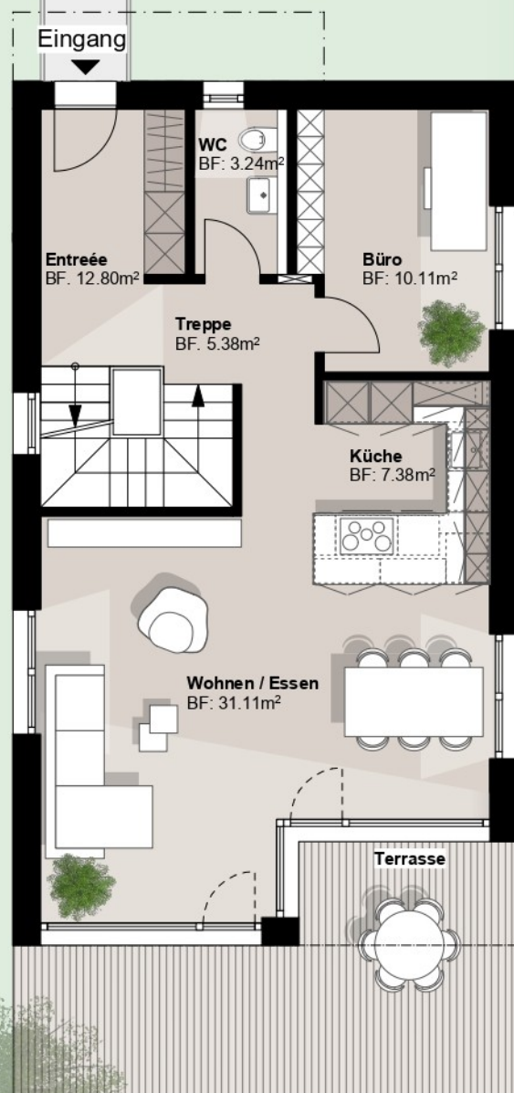
Haus Nr. 16 Grundriss EG (5.5 Zimmer EFH) Brutto-Geschossfläche = 86.50m² + Terrasse 20.81m² 1:100
