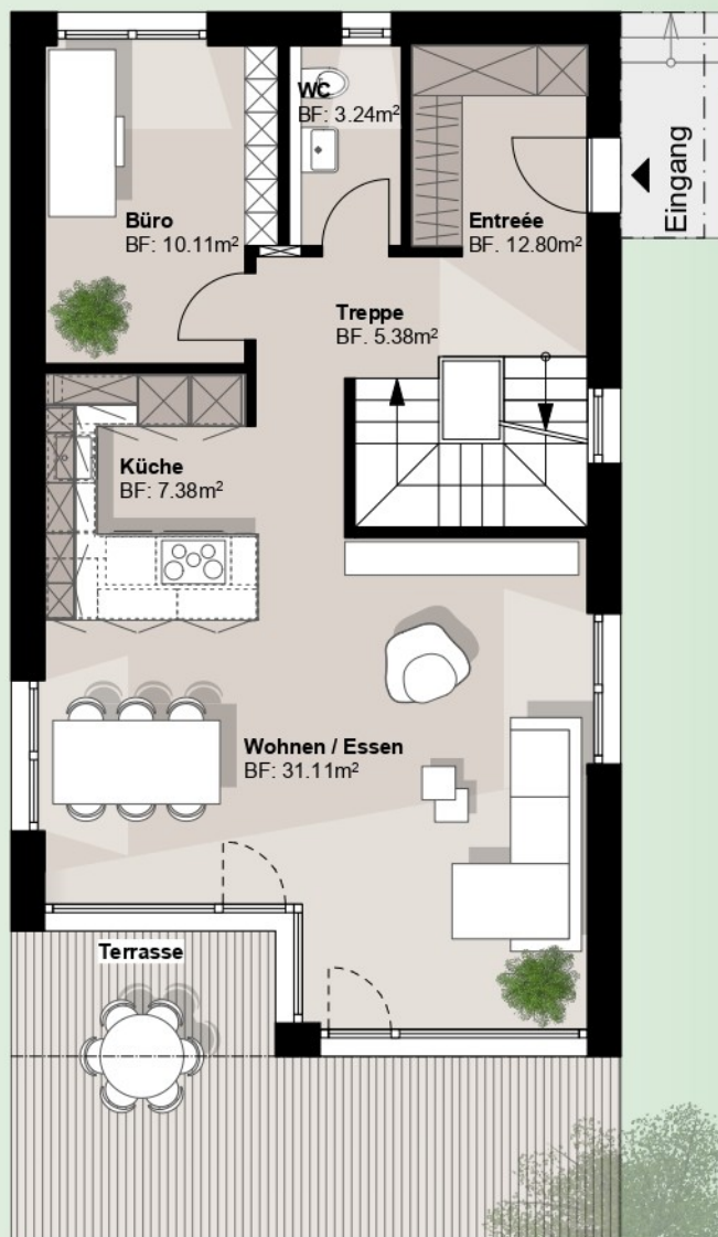
Haus Nr. 14 Grundriss EG (5.5 Zimmer EFH) Brutto-Geschossfläche = 86.50m² + Terrasse 20.81m² 1:100
