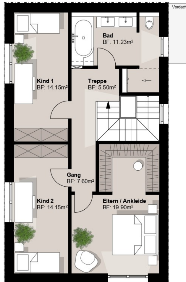
Haus Nr. 14 Grundriss OG, (5.5 Zimmer EFH) Brutto-Geschossfläche = 91.25m² 1:100
